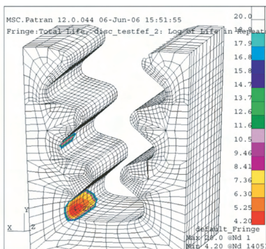
Rys. 6. Wyniki analizy zmęczeniowej S-N (trwałość zmęczeniowa poszczególnych stref modelu opisana jest w formie wykładniczej); minimalna trwałość zmęczeniowa dysku równa jest 10^{4.20} zaś łopatkki 10^{5.44} h pracy silnika
