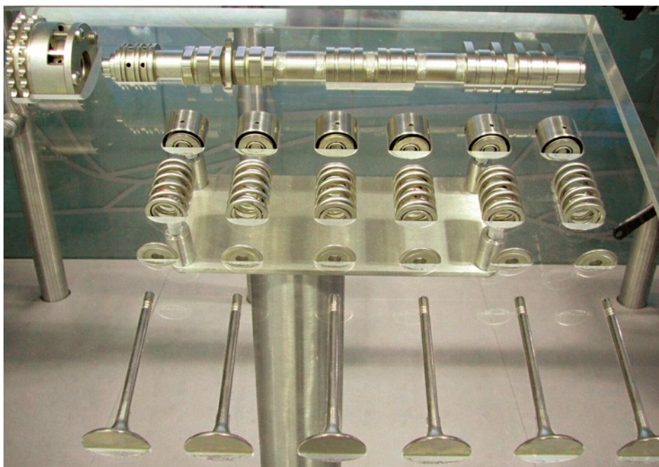
Rys. 21. Elementy składowe systemu zmiany wzniosu zaworów VarioCam silnika Porsche 3,6 dm 3 Bi-Turbo
