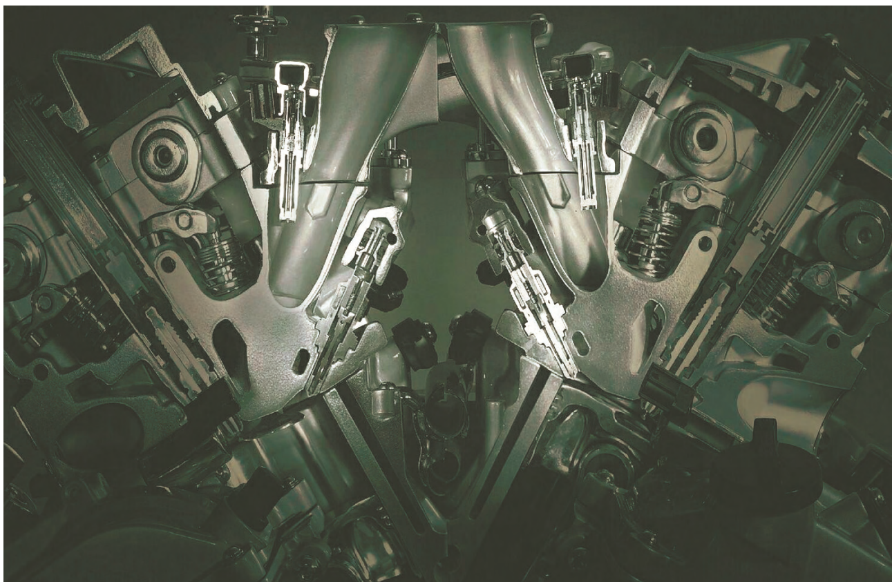
Rys. 22. Przekrój kanałów dolotowych i systemu spalania silnika 1UR-FSE samochodu Lexus LS 460
