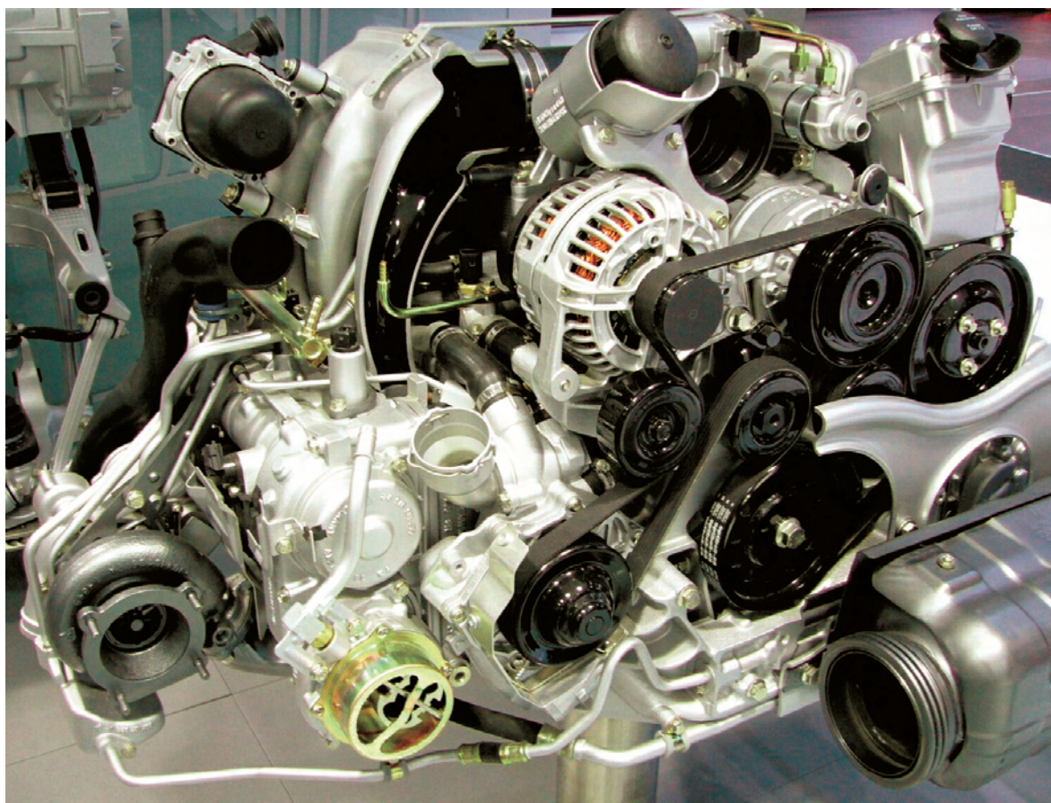
Rys. 19. Silnik typu bokser samochodu Porsche 3,6 dm 3 Bi-Turbo
