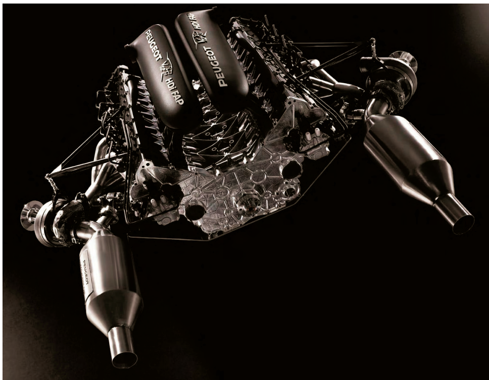
Rys. 7. Silnik o zapłonie samoczynnym V12 HDi koncernu PSA
