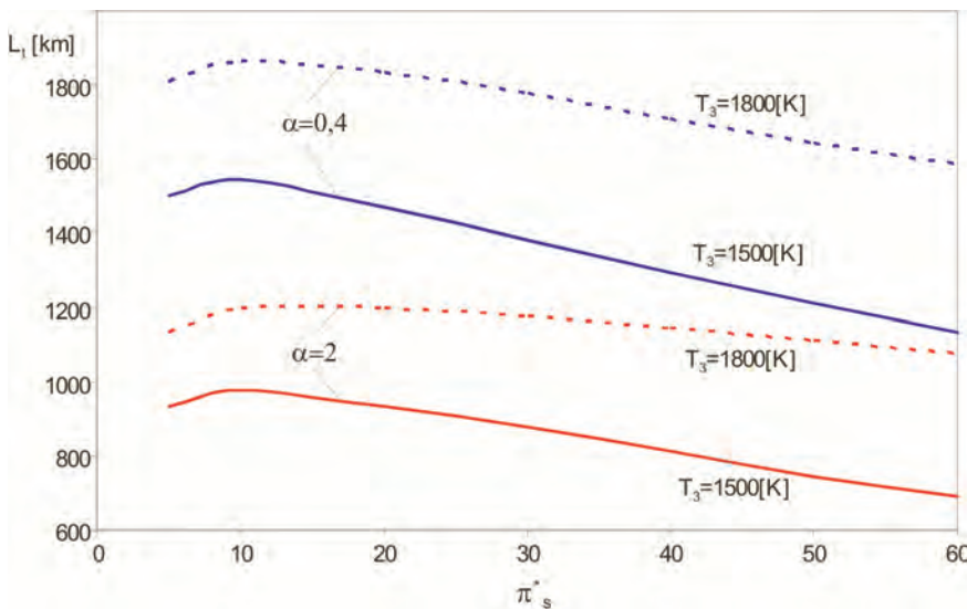
Rys. 12. Wpływ sprężu całkowitego silnika \pi_s^* , temperatury przed turbiną T_3^* , stopnia dwuprzepływowości a , na zmianę zasięgu teoretycznego L_1 ( Ma = 0,8 , H = 0 )
