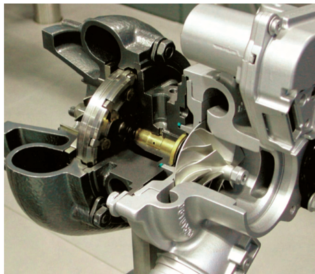
Rys. 20. Turbosprężarka silnika Porsche 3,6 dm 3 Bi-Turbo
