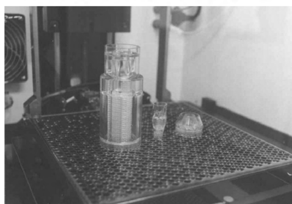
Rys. 3. Moduły wtryskiwacza – projekt komputerowy oraz po wykonaniu z żywicy epoksydowej metodą stereolitografii
