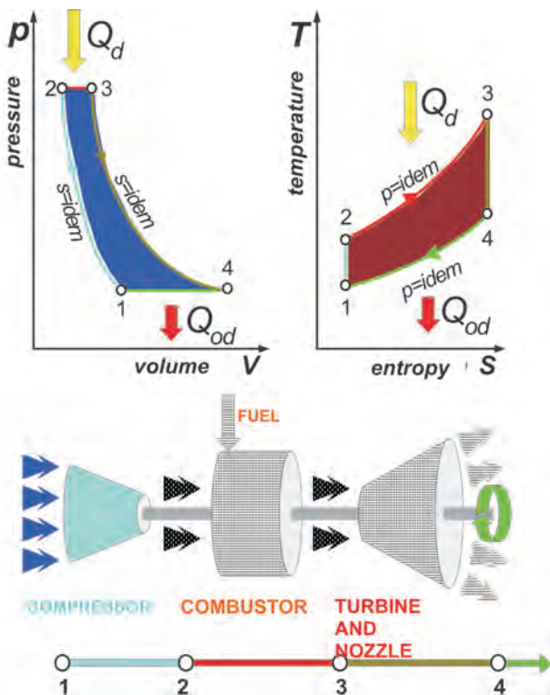
Rys. 7. Obieg Braytona i schemat turbinowego silnika odrzutowego
