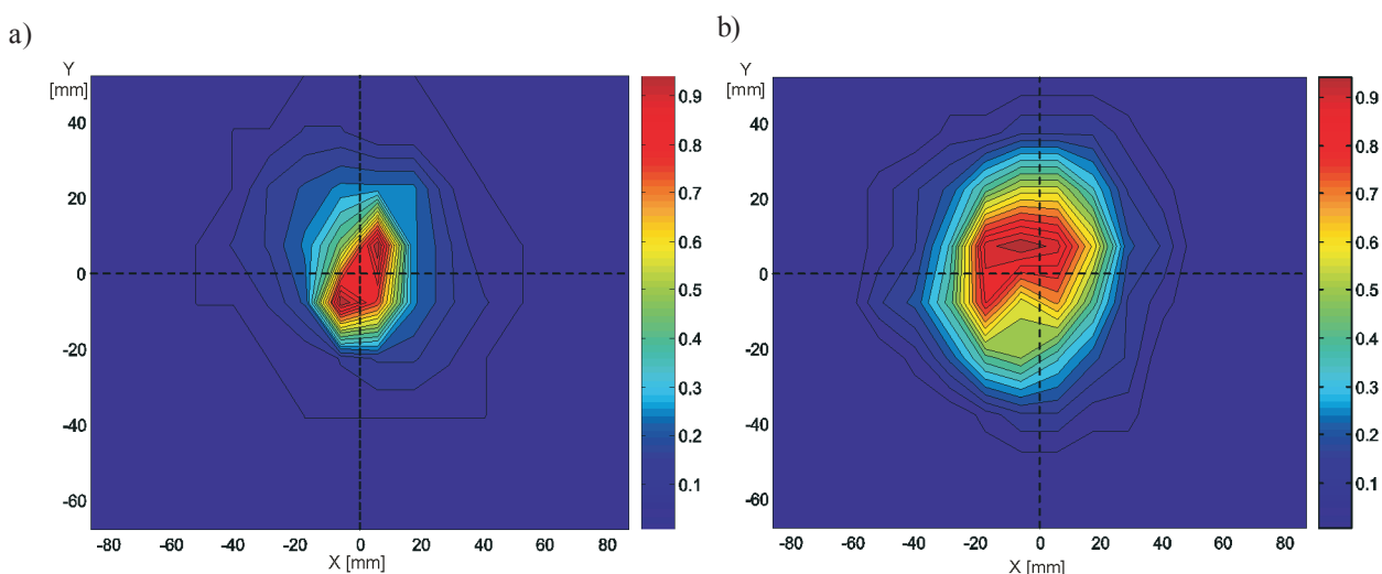
Rys. 12. Względny rozkład gęstości zraszania dla względnego wydatku wody 70% i względnego ciśnienia powietrza: a) 10%, b) 30% Fig. 12. Distribution of relative drops area for relative water flow rate 70% and relative air pressure: a) 10%, b) 30%
