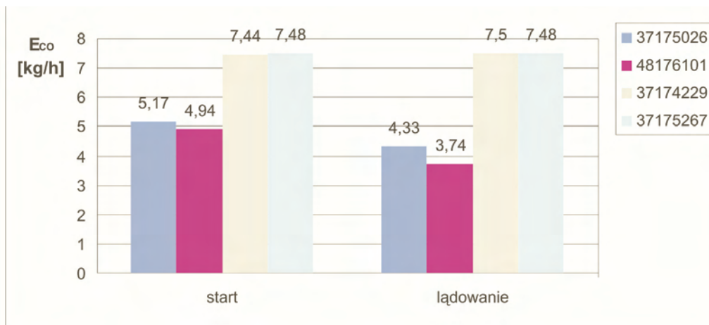
Rys. 11. Emisja godzinowa tlenku węgla w silnikach typu SO-3 dla startu i lądowania Fig. 11. Hourly emission of carbon monoxide in SO-3 engines for take-off and landing phases
