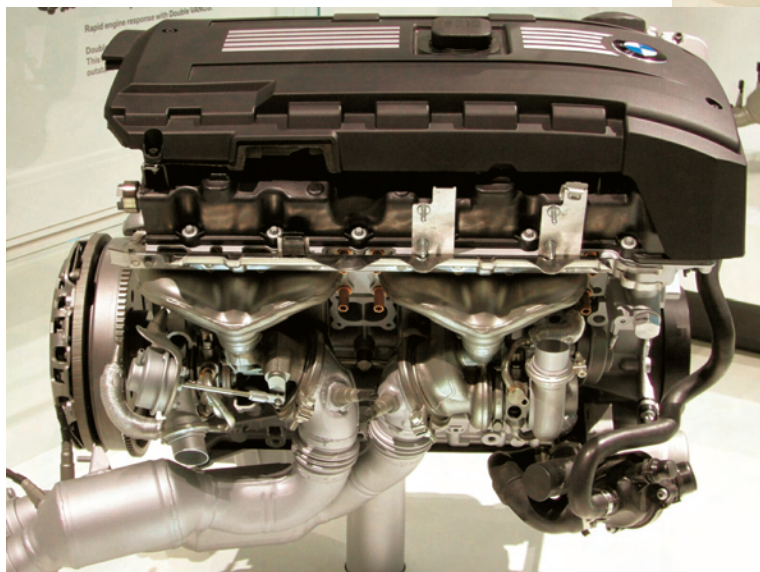
Rys. 15. Strona układu wylotowego silnika BMW 3,0 dm 3 Twin Turbo
