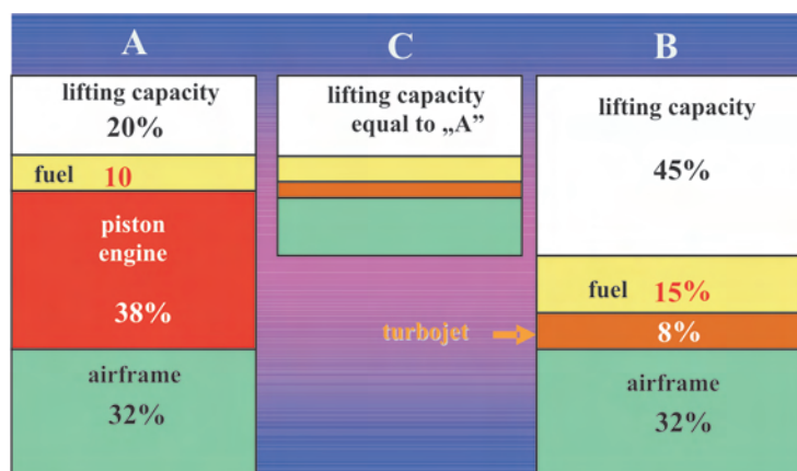
Rys. 20. Rozkład masy startowej samolotów myśliwskich przygotowanych do jednogodzinnego lotu z jednakową prędkością na wysokości 6000 m
