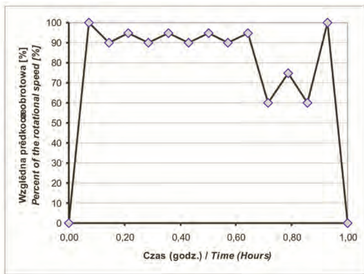
Rys. 5. Uproszczona historia obciążenia odpowiadająca godzinnej pracy silnika Fig. 5. Simplified load spectrum of turbine for 1-hours of engine operation
