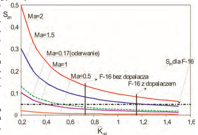
Rys. 3. Wpływ \overline{K_{sil}} na wartość S_{ZN} dla różnych warunków lotu (wyrażonych liczbą Ma )
