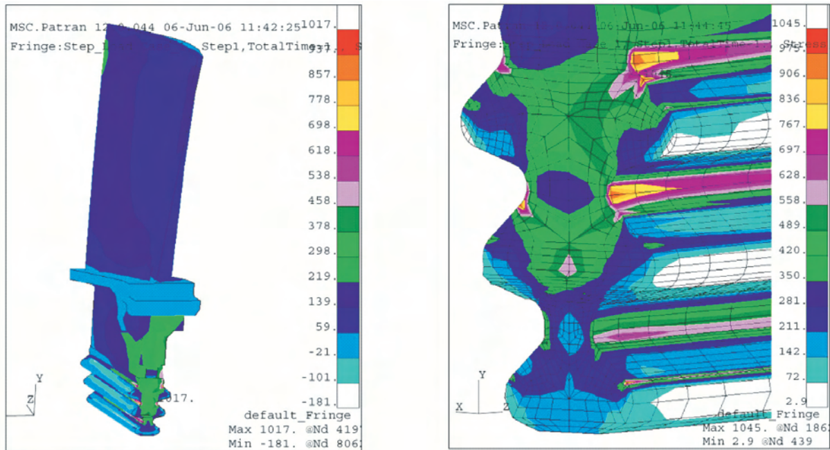
Rys. 4. Rozkład naprężeń maksymalnych głównych ( s_1 ) (a) oraz zredukowanych według hipotezy Hubera-Misesa-Hencky'ego (b) dla łopatki obracającej się z prędkością obrotową 14000 obr/min
