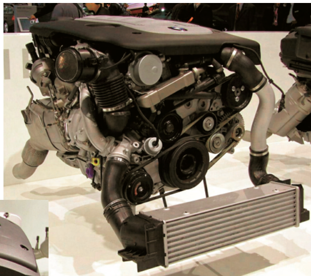
Rys. 17. Silnik o zapłonie samoczynnym BMW 3,0 dm 3 Variable Twin Turbo
