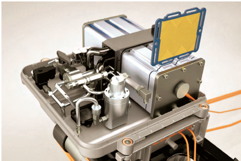
Rys. 5. Ogniw paliwowe GENEPAAC 20 koncernu PSA
