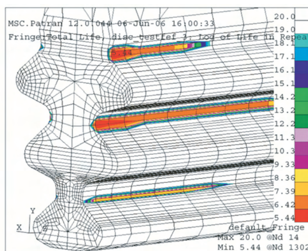
Rys. 6. Wyniki analizy zmęczeniowej S-N (trwałość zmęczeniowa poszczególnych stref modelu opisana jest w formie wykładniczej); minimalna trwałość zmęczeniowa dysku równa jest 10^{4.20} zaś łopatkki 10^{5.44} h pracy silnika
