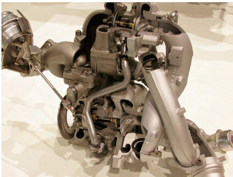
Rys. 16. Układ doładowania silnika o zapłonie samoczynnym BMW 3,0 dm 3 Variable Twin Turbo
