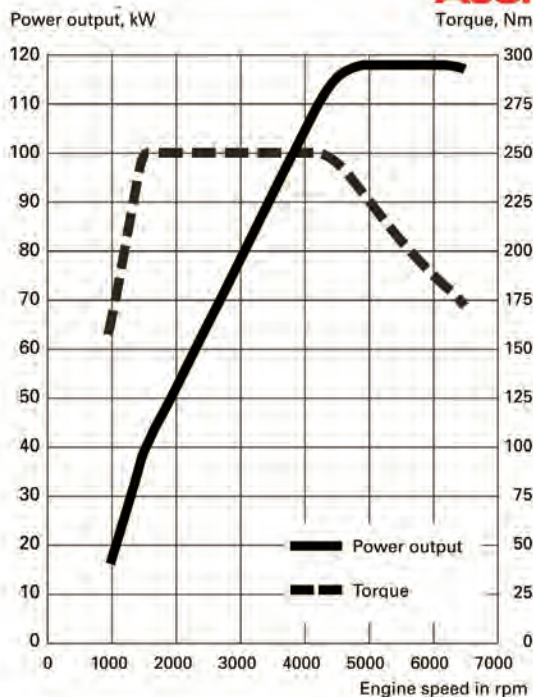
Rys. 13. Charakterystyka prędkościowa silnika 1,8 TFSI
