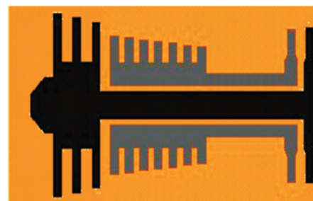
Rys. 24. Schemat układu wirników dwuprzepływowego silnika turbinowego F404-GE-400 Fig. 24. A scheme of the two rotors mechanism of the turbofan F404-GE-400
