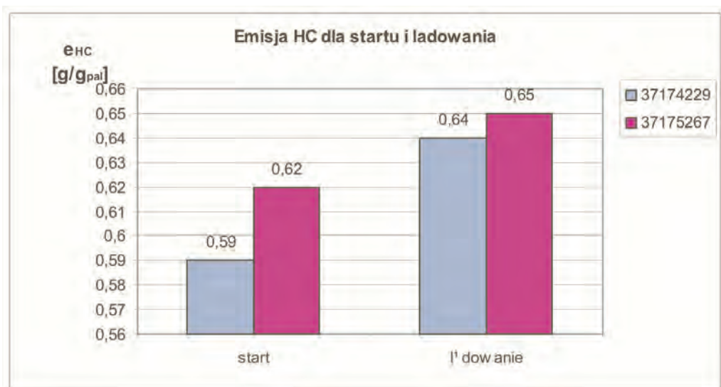
Rys. 14. Emisja węglowodorów z jednostki spalonego paliwa w silnikach typu SO-3 dla startu i lądowania Fig. 14. The hydrocarbons emission from unit of consumed fuel in engines SO-3 for phase take-off and landing
