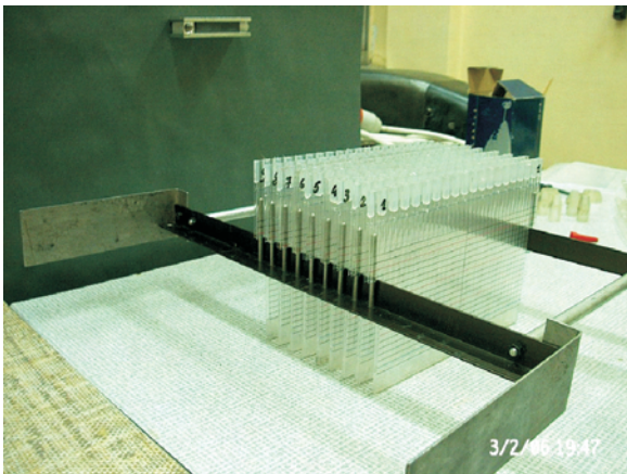
Rys. 7. Sonda grzebieniowa Fig 7. Comb probe
