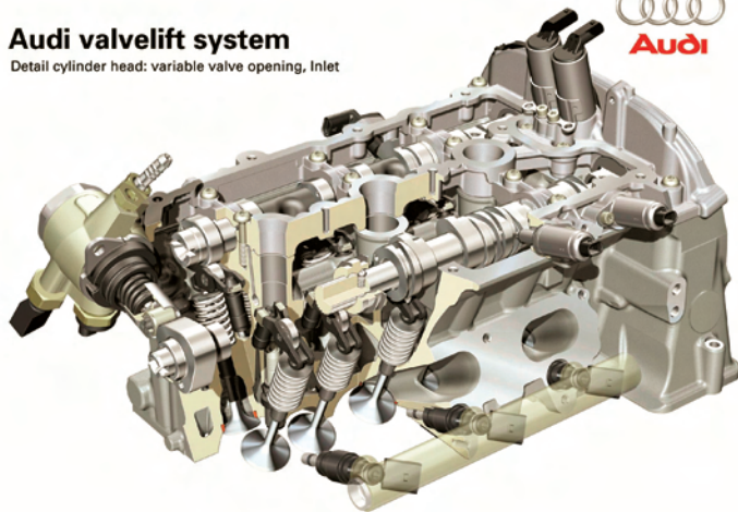
Rys. 9. Przekrój głowicy silnika Audi 2,8 FSI z systemem Valvelift
