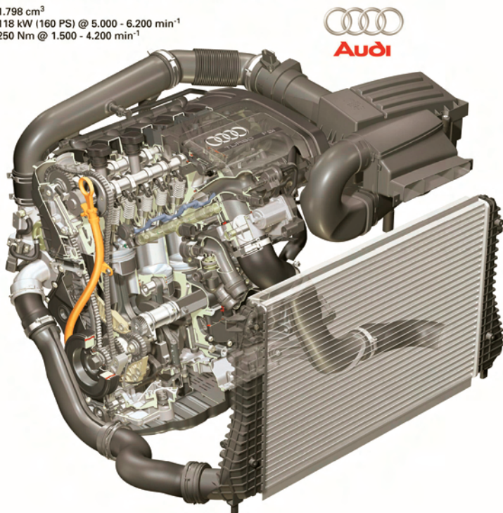
Rys. 12. Przekrój silnika 1,8 TFSI
