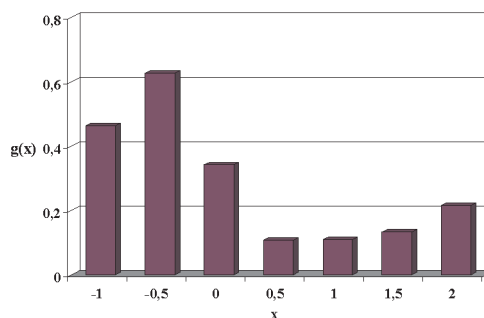
Fig. 9. The probability density g(x) of the standardized specific road emission of particulate matter b_{PMs} from passenger vehicle engines Rys. 9. Gęstość prawdopodobieństwa g(x) standaryzowanej emisji drogowej cząstek stałych b_{PMs} z silników samochodów osobowych
