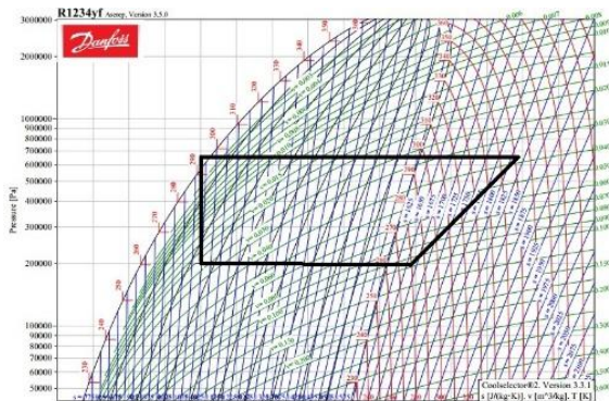
Fig. 10. Linde cycle
