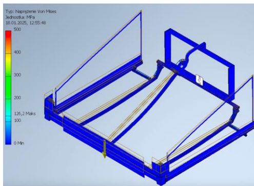
Fig. 11. Von Mises stresses – gravity
